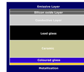
CEMタイプKBL表面構造の断面図
